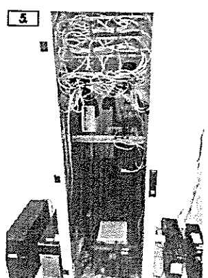
5. Kábelfejtés rendezészekrényben, optikai kábeltartók a szekrény hátuljában elhelyezve
